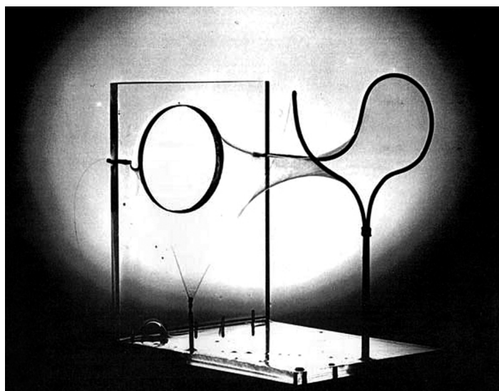
Imaxe de ensaio no Institut für leichte Flächentragwerke. Universidad de Stüttgart
